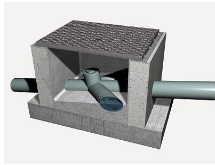
Exemple de registre de col·lector mitjançant arqueta
